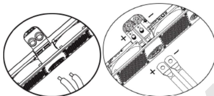
Модель 1.5кВт
