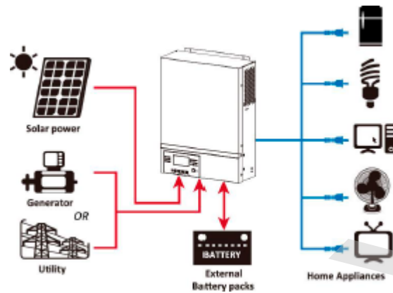
Рис. 1. Гибридная система энергоснабжения
