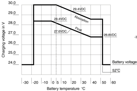
Schéma 11. Compensation en température sur les modèles CX24xx
